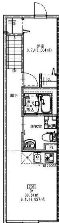
住戸面積 205号室 30.84㎡
