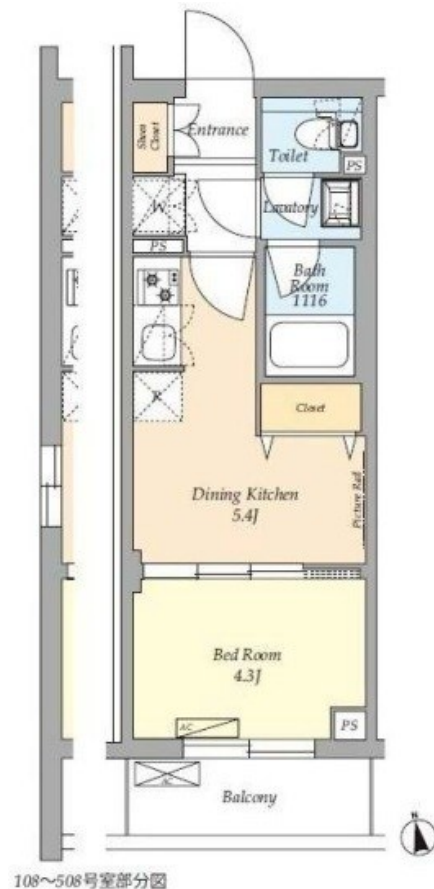
108〜508号室部分図
